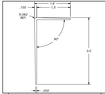
D*80752 L-Trim
