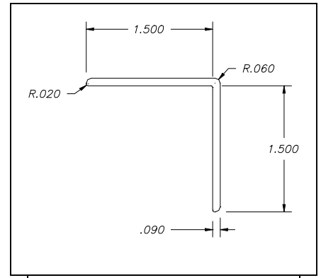
R*1171 L-Trim
